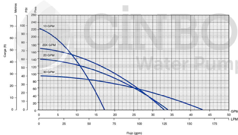
CURVA DE RENDIMIENTO DE LA FAMILIA SERIE C1
