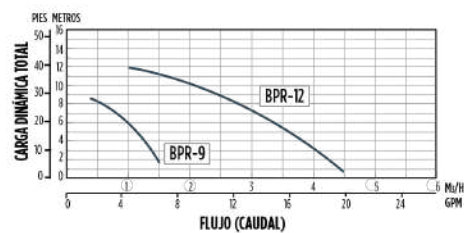
CURVA DE RENDIMIENTO DE LA FAMILIA SERIE BPR
